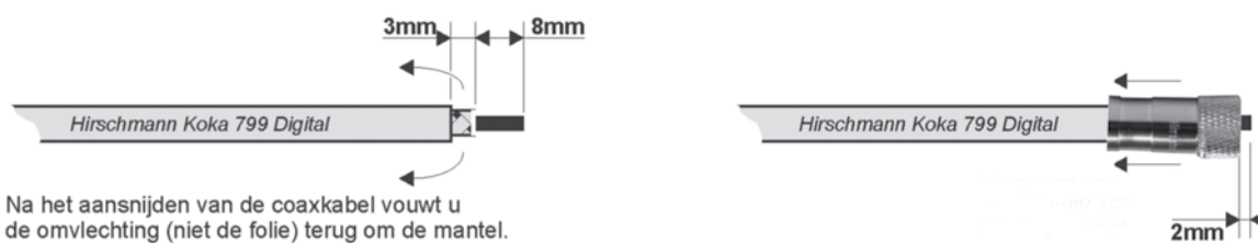
F connector POFC 070 t.b.v. KOKA 799 en COAX 12
