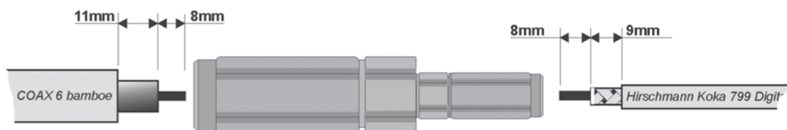
Koppeling KVB C6/C12 t.b.v. COAX 6 Bamboe kabel naar KOKA 799 of COAX 12 kabel
