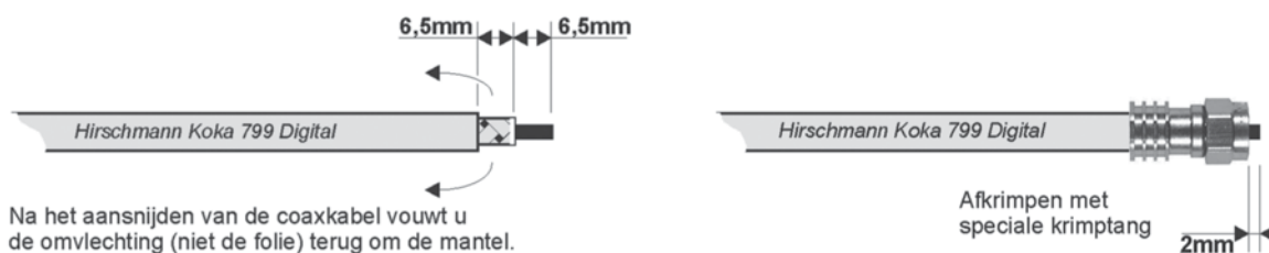
F connector SFC 012 t.b.v. KOKA 799 en COAX 12
